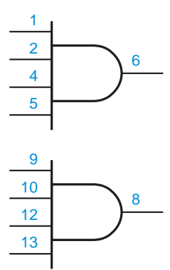
74x21
