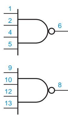
74x20
