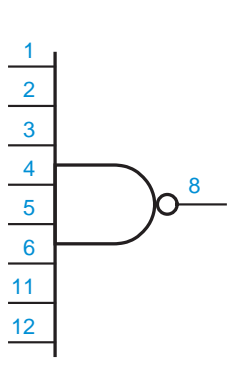
74x30
