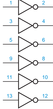
74x04
