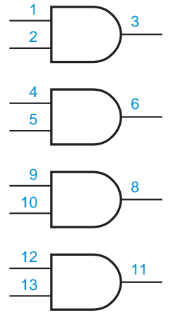
74x08
